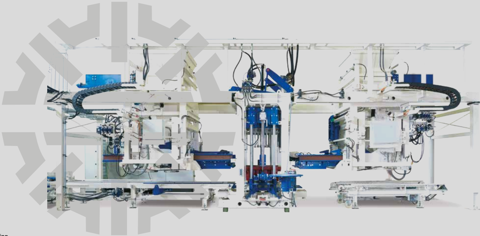
TTT Transport der Produkte auf Paletten Транспортировка изделий на поддонах
